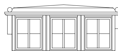
TAKKUPA TYP E3 ELEVATION - FRAMSIDAN
