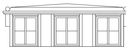
TAKKUPA TYP E2 ELEVATION - FRAMSIDAN
