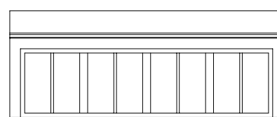
TAKKUPA TYP C ELEVATION - FRAMSIDAN
