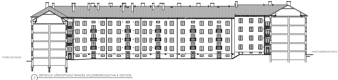
2. BEFINTLIG GÅRDSFASAD BAKOM GYLLENBORGSGATAN & SEKTION
