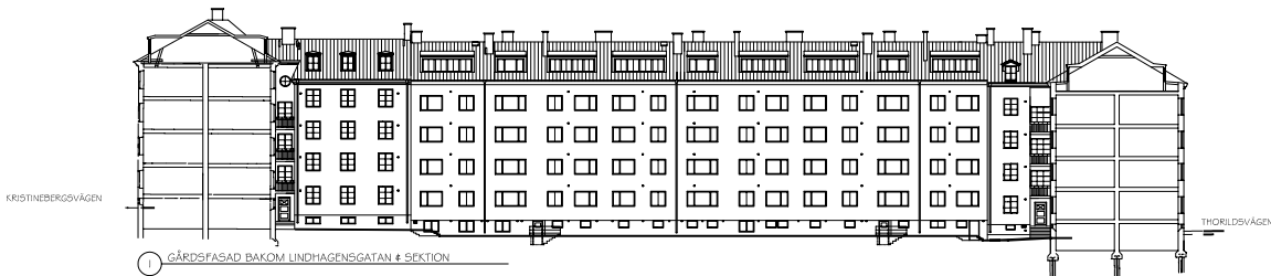
1. GÅRDSFASAD BAKOM LINDHAGENSGATAN & SEKTION
