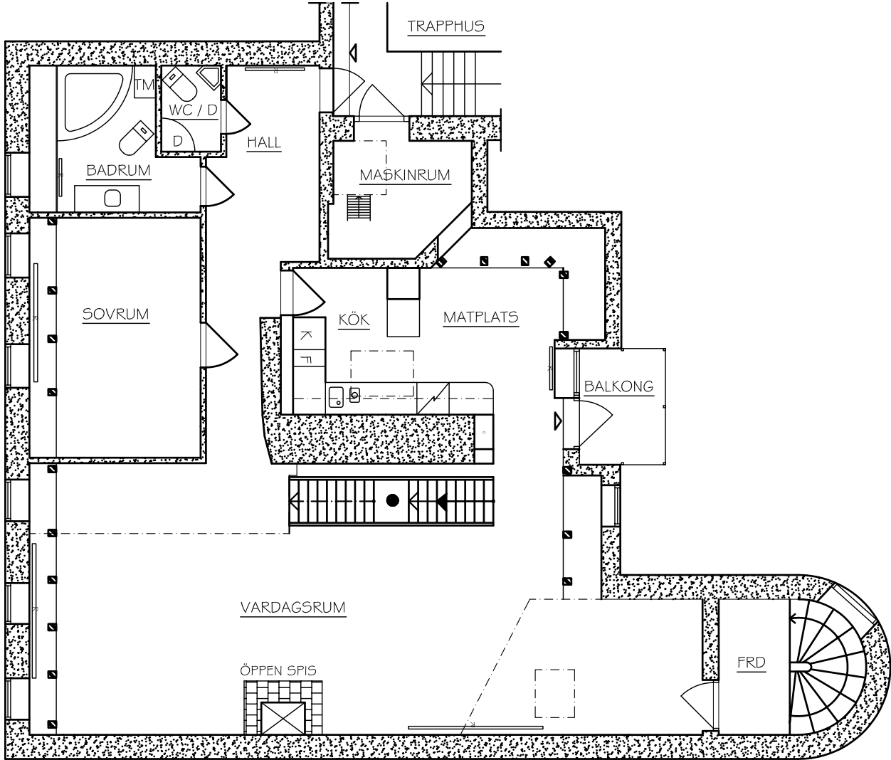
BEFINTLIG ENTRÉPLAN
