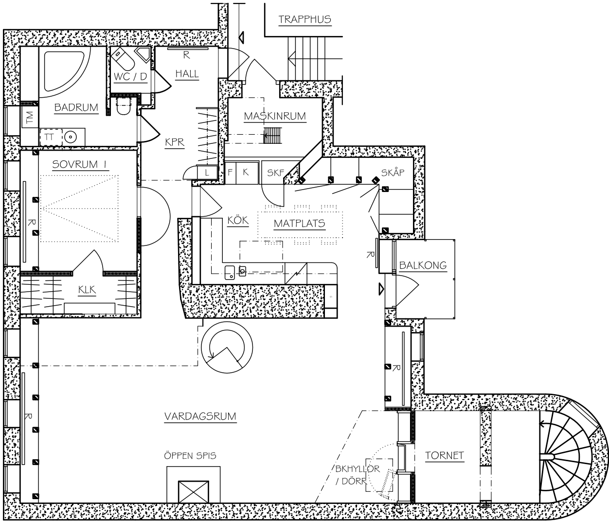
ENTRÉPLAN FÖRSLAG
